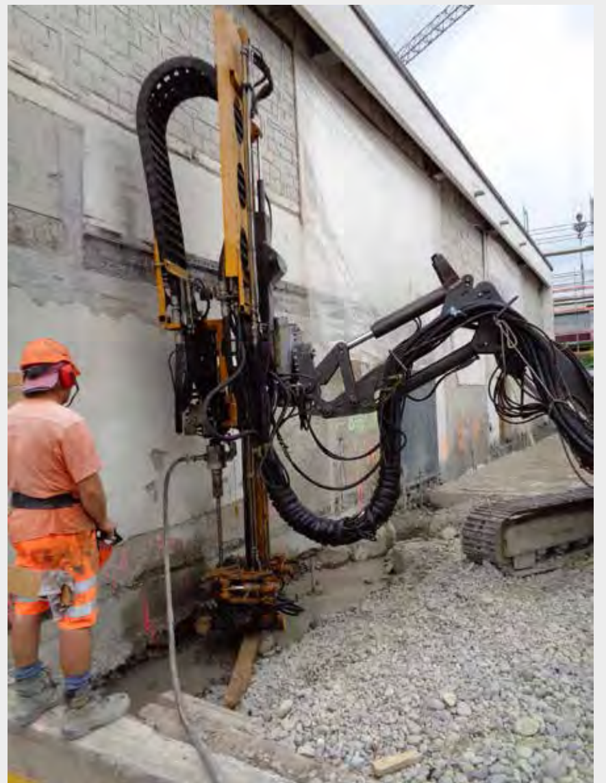
Die Bohrmaschine wurde für die Vorbereitung der zusätzlichen Pfählungen eingesetzt.
